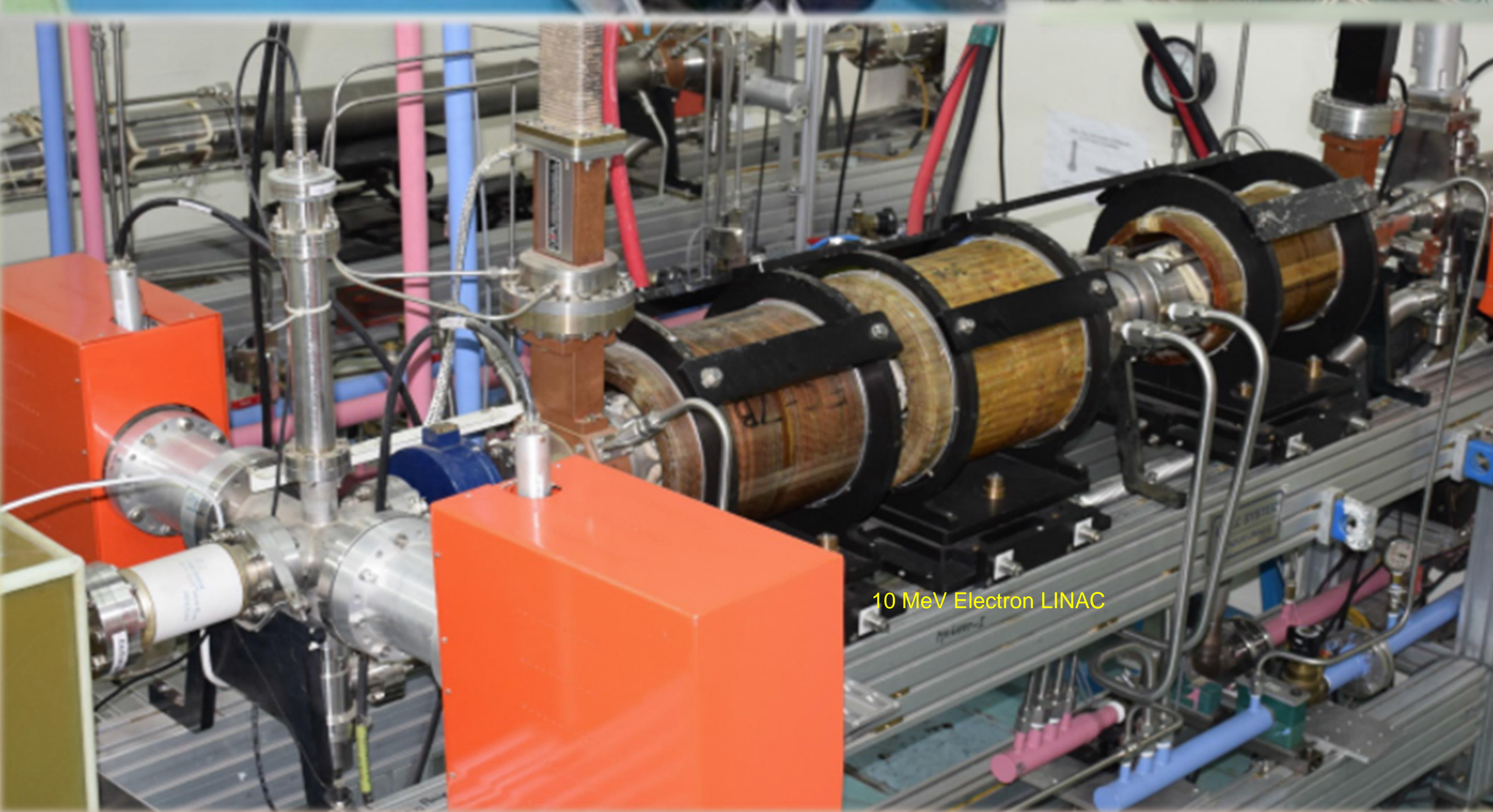
H-Ion Source and LEBT
